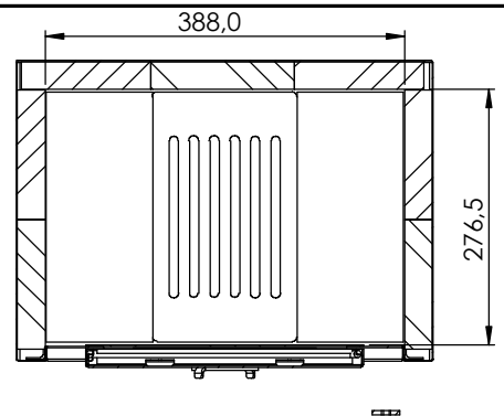
SECTION B-B SCALE 1 : 6
