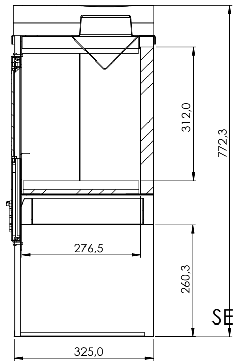
SECTION B-B SCALE 1 : 6
